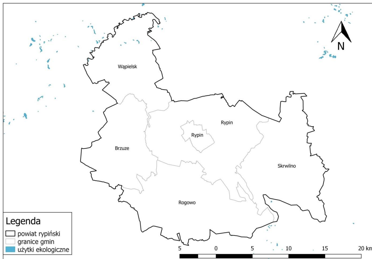
Mapa 16. Użytki ekologiczne w powiecie rypińskim
