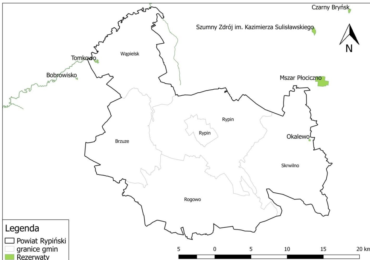
Mapa 13. Rezerwaty przyrody na terenie powiatu rypińskiego
