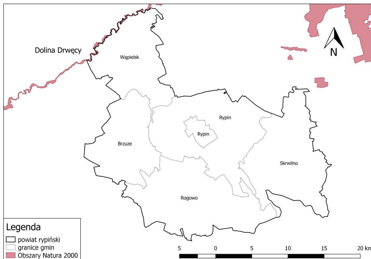
Mapa 15. Obszary Natura 2000 na terenie powiatu rypińskiego
