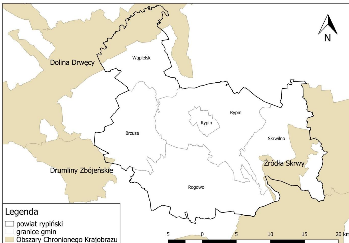
Mapa 14. Obszary Chronionego Krajobrazu na terenie powiatu rypińskiego
