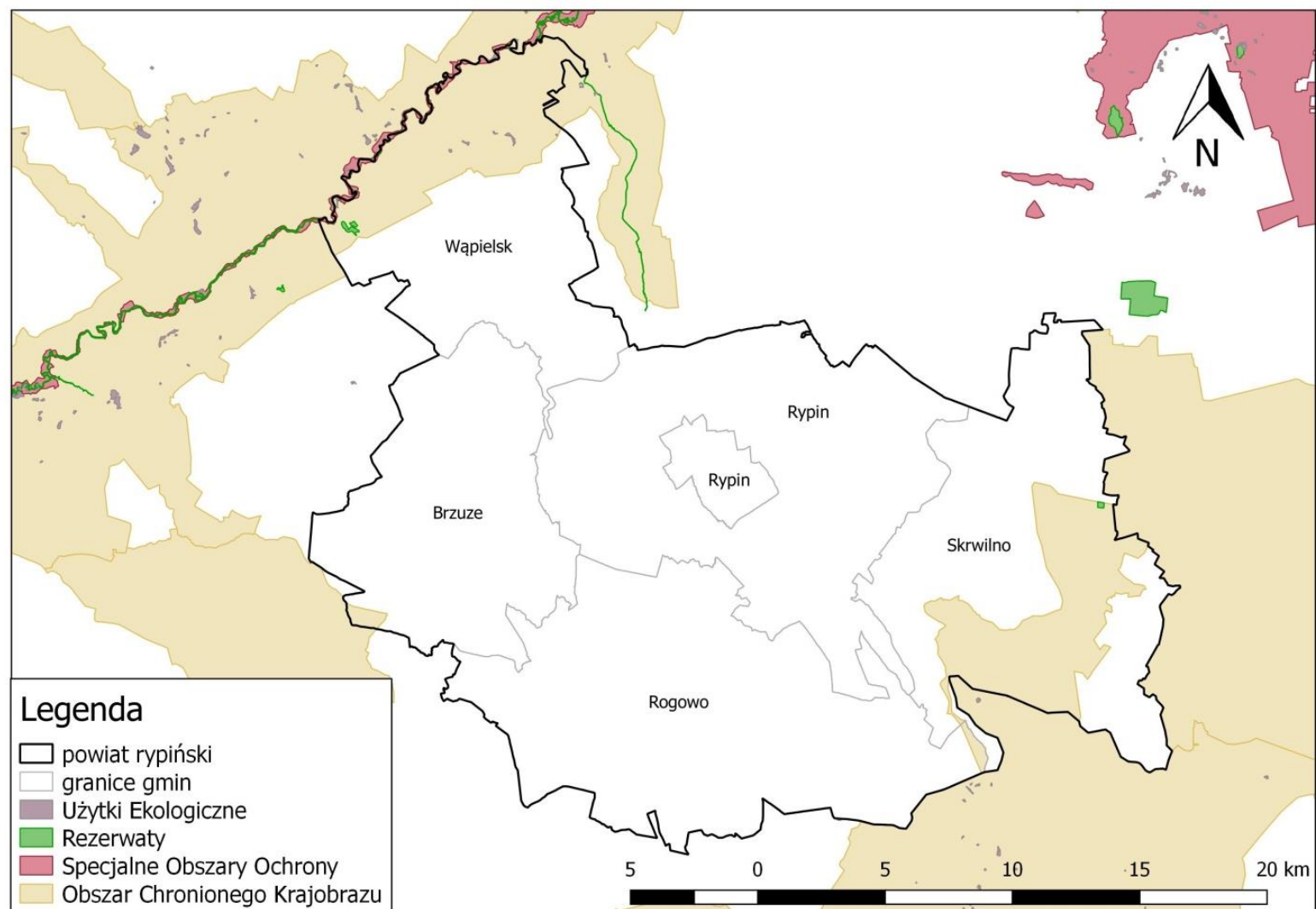
Mapa 12. Formy ochrony przyrody na terenie powiatu rypińskiego
